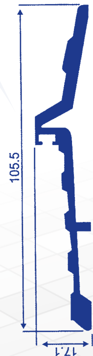
71605 (1.139 Kg/M)
